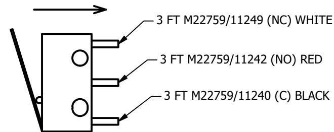
MDG13B1LA- MICROSWITCH
